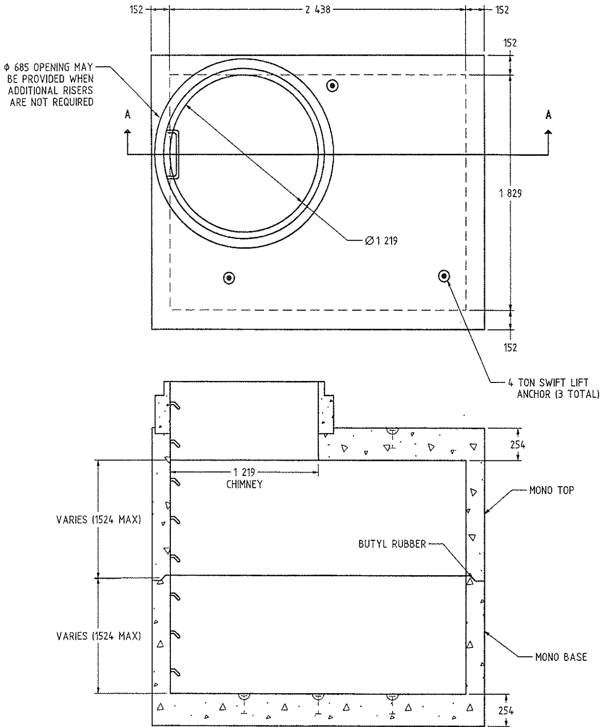
SECTION A-A
